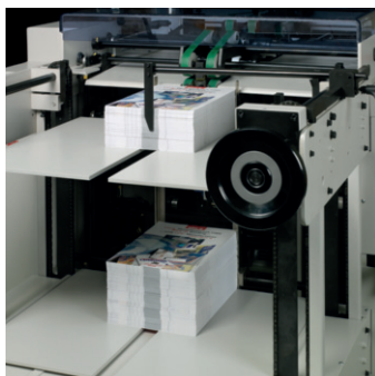
High pile feeder Carga en continuo Margeur haut de pile Hochstapel-Anleger
