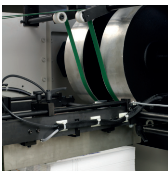
Sheet turnover Salida de las hojas Tambour de retournement Wendetrommel
