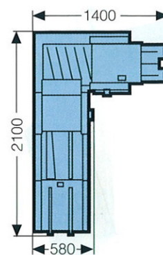
Multipli 35/2/4 PBA
