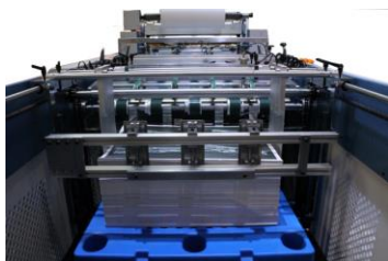
Margeur haut de pile / Sortie haut de pile avec taquage Séparation pneumatique
